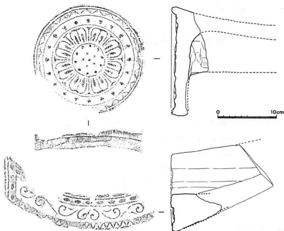
第2図 中ノ島遺跡出土軒丸・軒平瓦拓影・実測図
