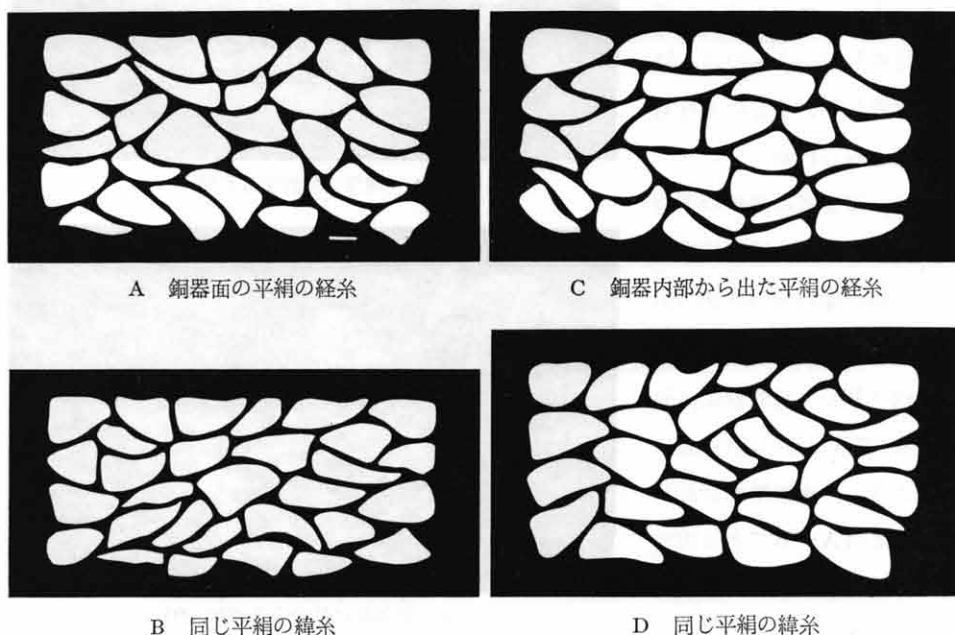
第3図 カジャ古墳出土の平絹の繊維断面転写図 (scale: 5 \mu 拡大率はA-Dに共通) (個々の断面転写図を無秩序に並べたもの)
