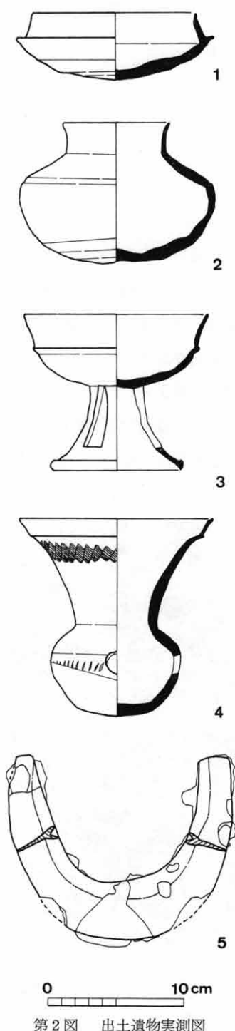
第2図 出土遺物実測図
