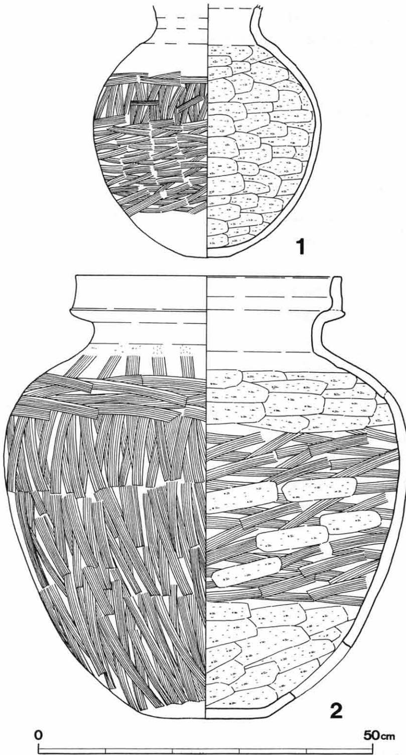
第3図 出土遺物実測図
