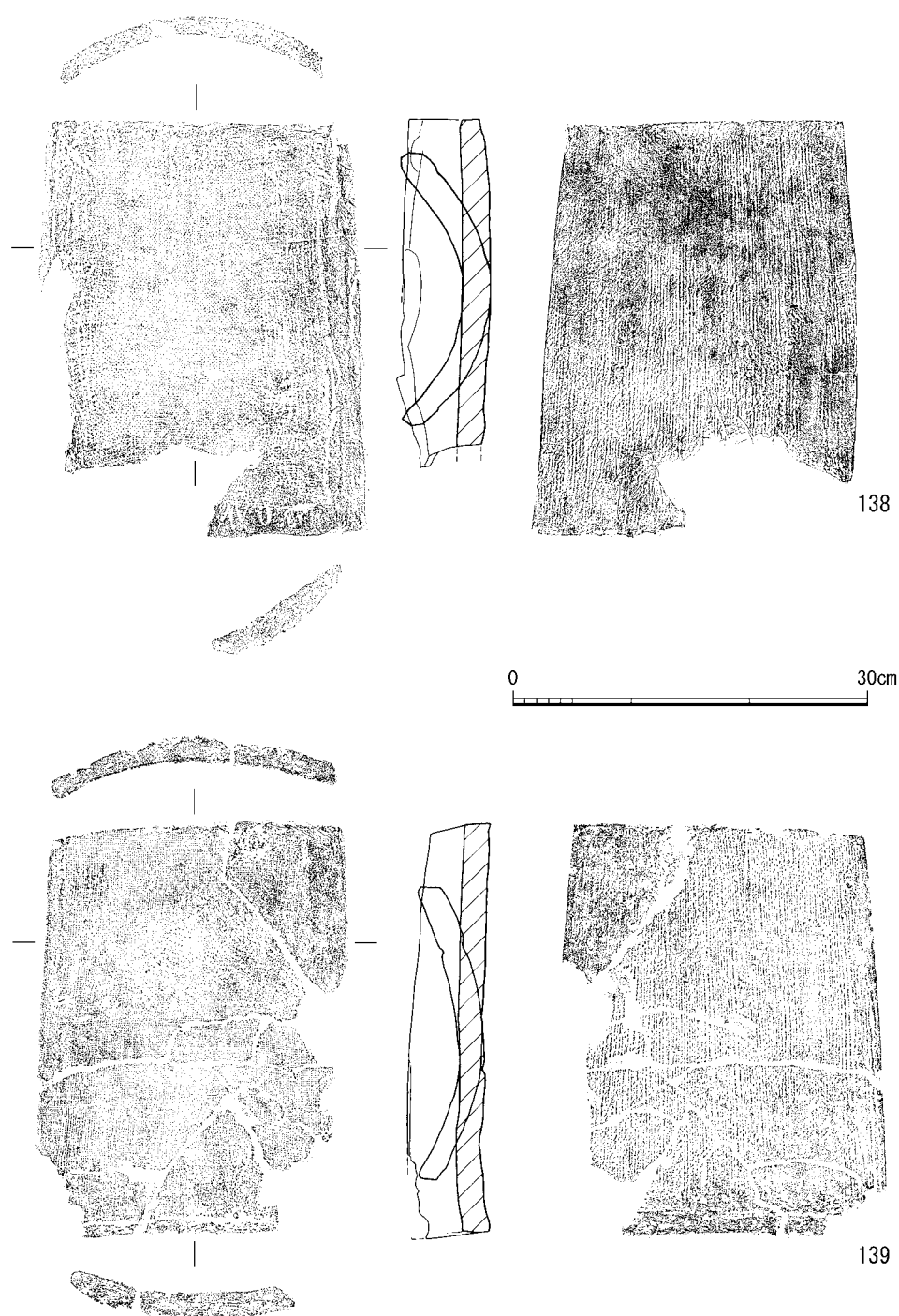
第55図 5号窯出土平瓦実測図2 隔壁
