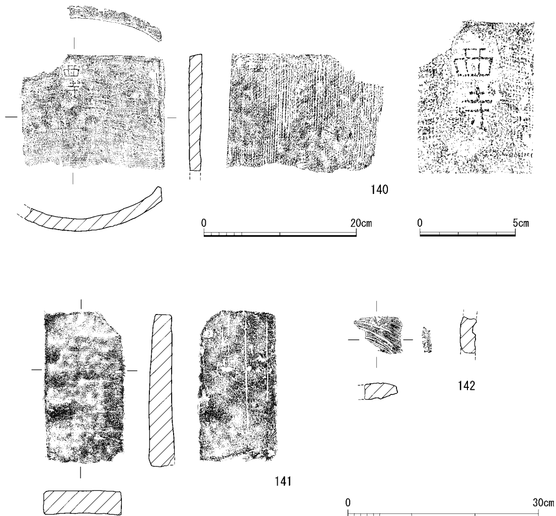
第56図 「西寺」銘瓦・塼・鴟尾実測図
