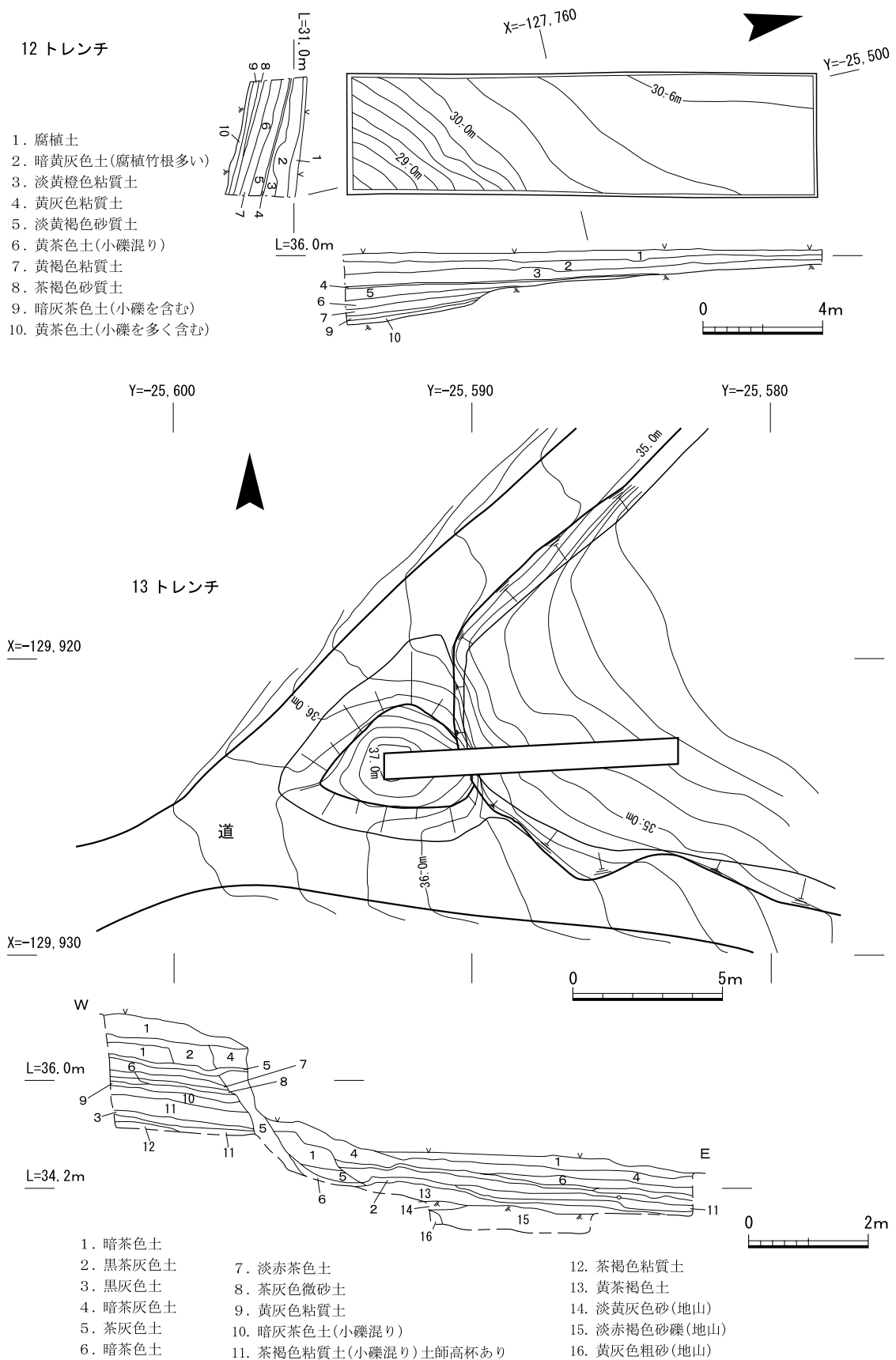
第61図 12・13トレンチ実測図
