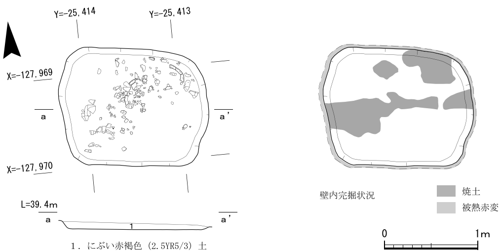
第17図 土師器焼成坑 S Y 45実測図
