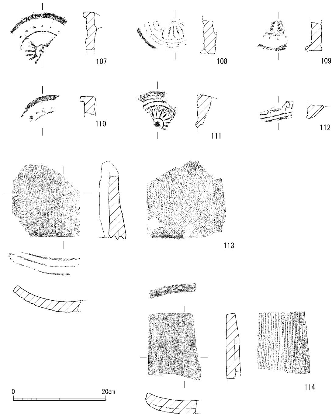
第44図 その他の遺構出土軒瓦実測図
