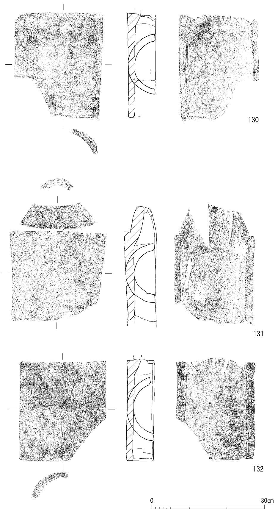
第52図 5号窯出土丸瓦実測図1 分焰柱
