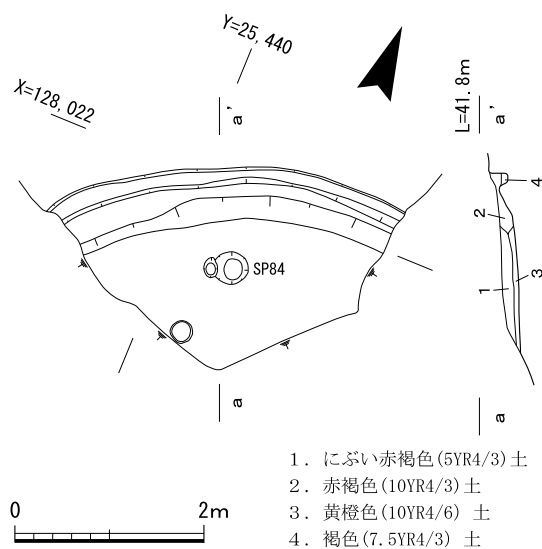
第10図 竪穴建物 S H35実測図
