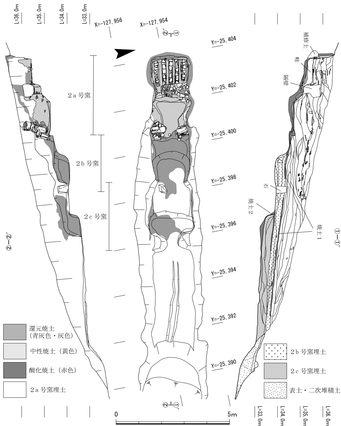
第33図 2号窯実測図
