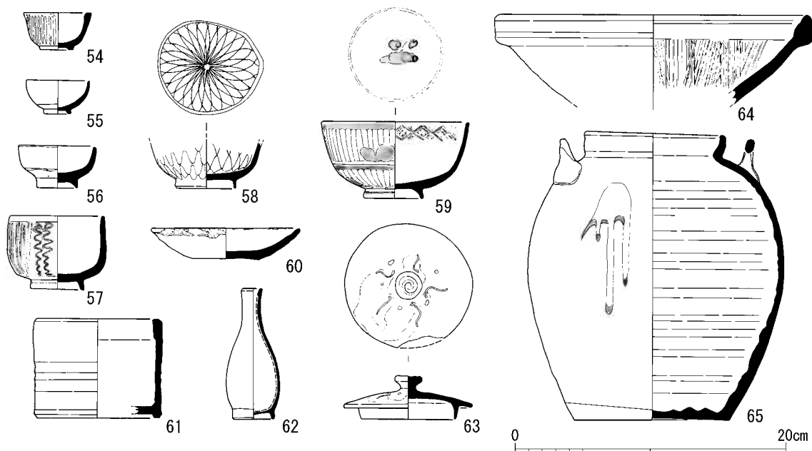
第28図 出土遺物実測図7(S K 32)
