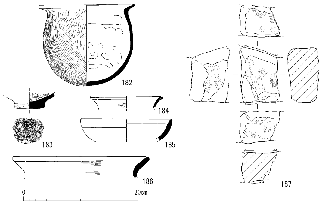
第67図 出土遺物実測図3
