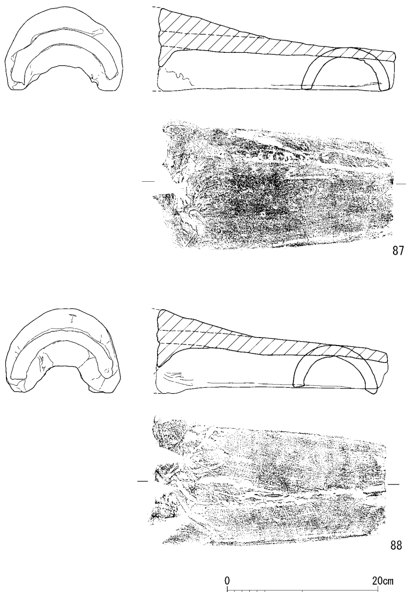
第41図 2号窯出土軒丸瓦実測図2
