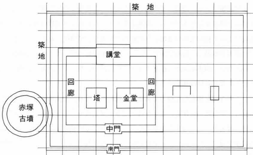
第2図 平川廃寺50尺方格伽藍配置計画図(1/2,000) (『城陽市埋蔵文化財調査報告書』第3集より再トレースした。)
