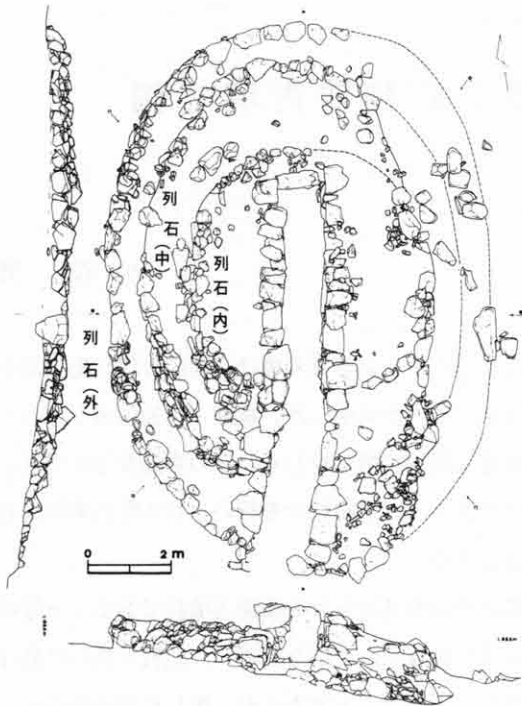
第2図 兵庫県八鹿町箕谷3号墳(1/180)
