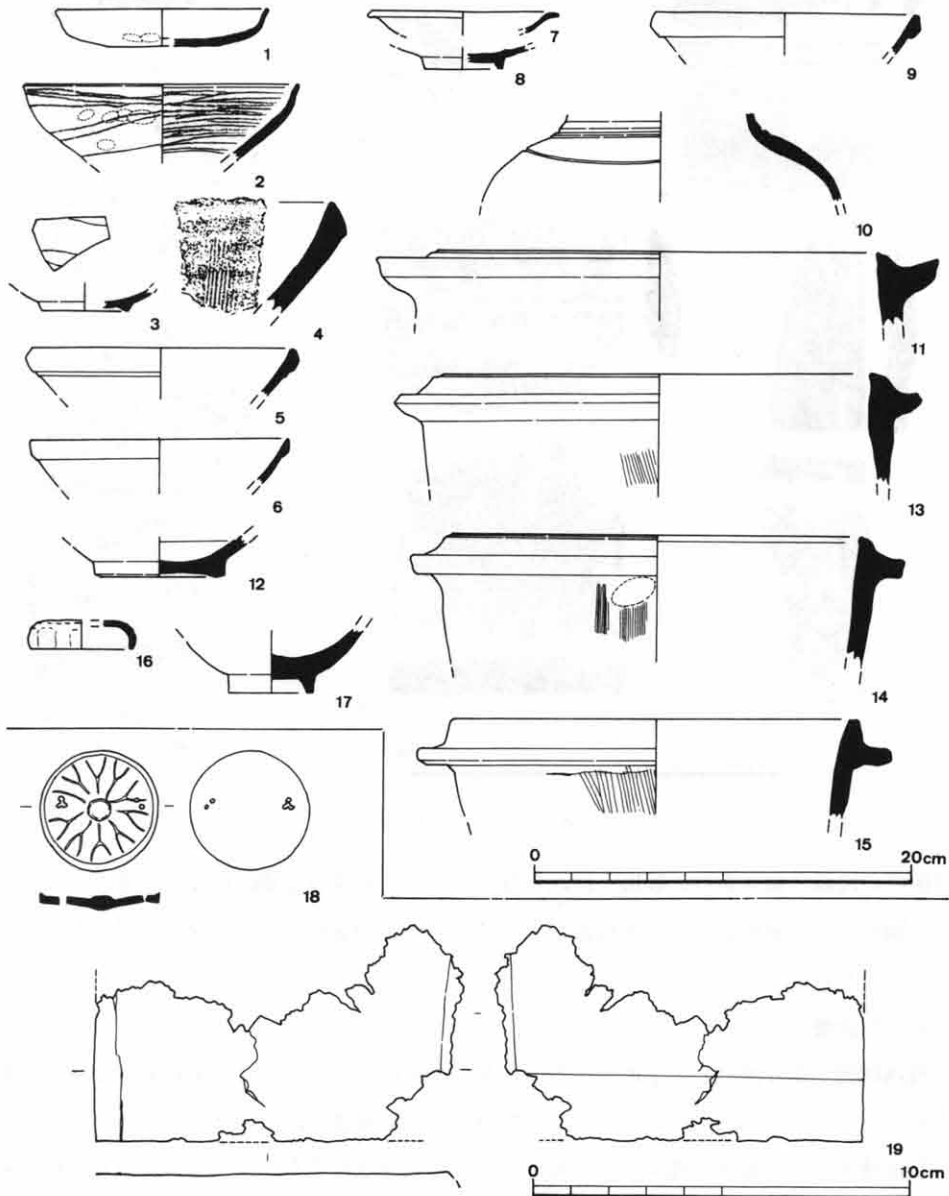
第4図 土器及び金属器実測図 (1～6はS D01、7～11はS D02、他は包含層)
