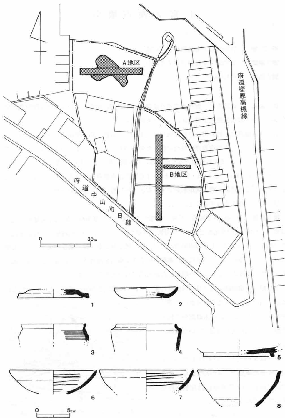
第2図 調査地位位置図及び出土遺物実測図
