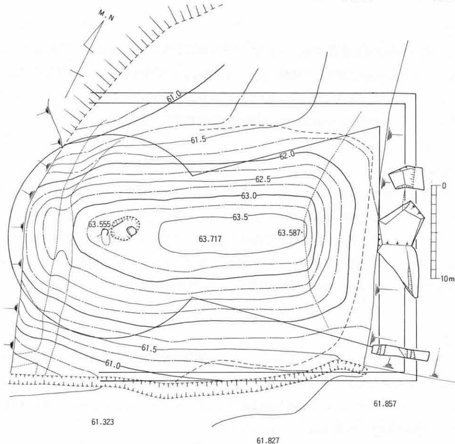
第3図 石神1号墳墳丘測量図
