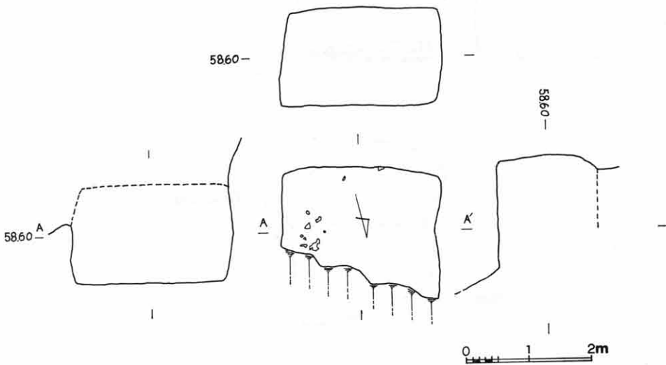
第4図 1号実測図
