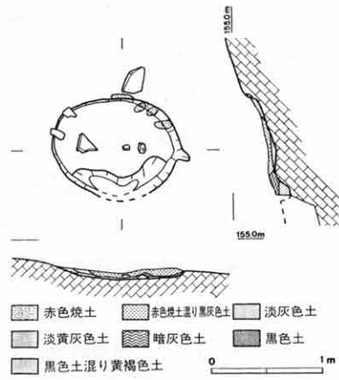
第2図 円形焼土壇実測図
