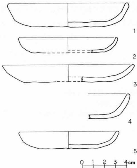
第6図 遺物 実測図
