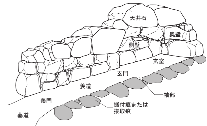
第3図 横穴式石室模式図
