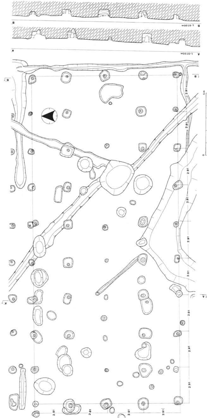
S B 301平面图
